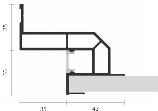
Schattenfugenprofil für Trockenbaudecken mit Trockenbauplatte in 12,5 mm Stärke
