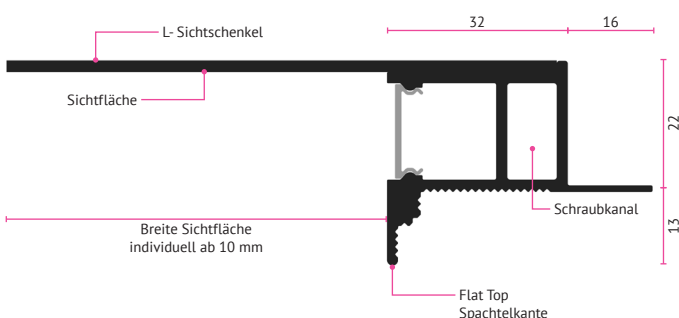
Schattenfugenprofil Individual mit Sichtschenkel gerade aus Trockenbauplatte
