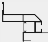
Schattenfugenprofil Standard
